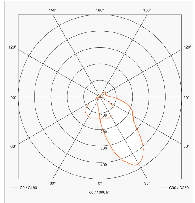
Optique Asymétrique : ASY - 2 Rendement 91 %
