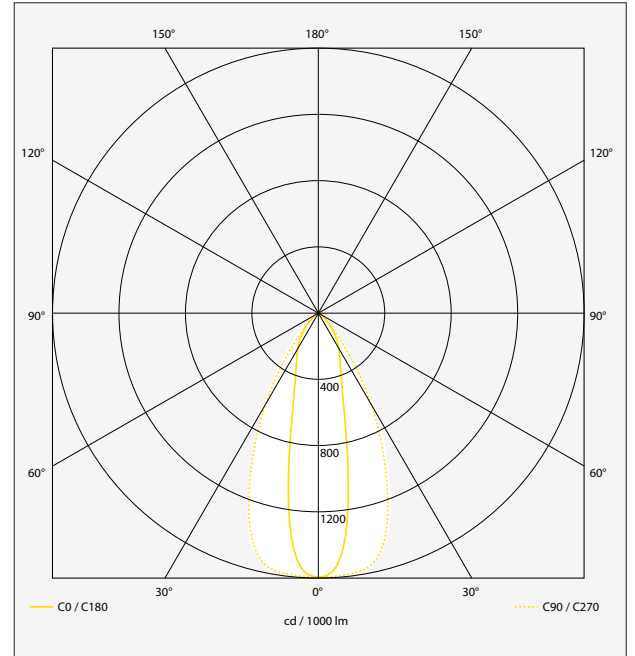
Elliptical LOR 96,5 %
