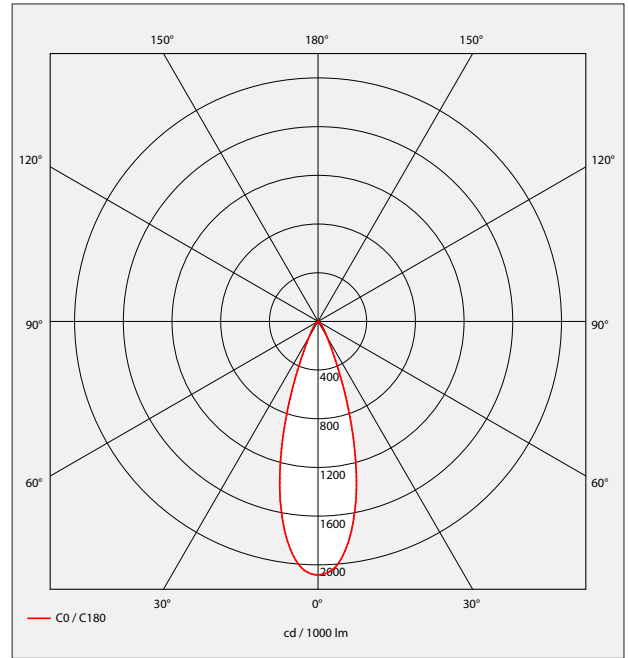
Faisceau 33° Rendement 75%
