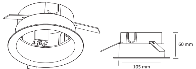
XTSA 71 : Boitier d'encastrement pour le GA 70
