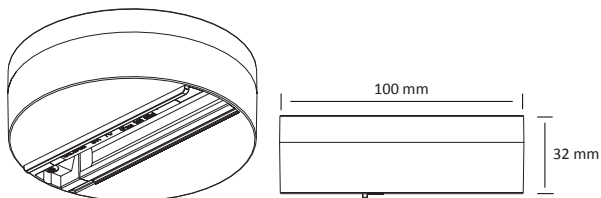
XTSA 67S : Adaptateur pour prise de courant
