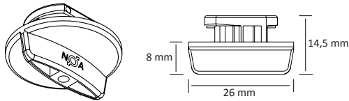
GA 69 : Adaptateur 3 Allumages avec tenue au poids de 5 Kg
