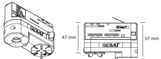
XTSA 71 : Boitier d'encastrement pour le GA 70
