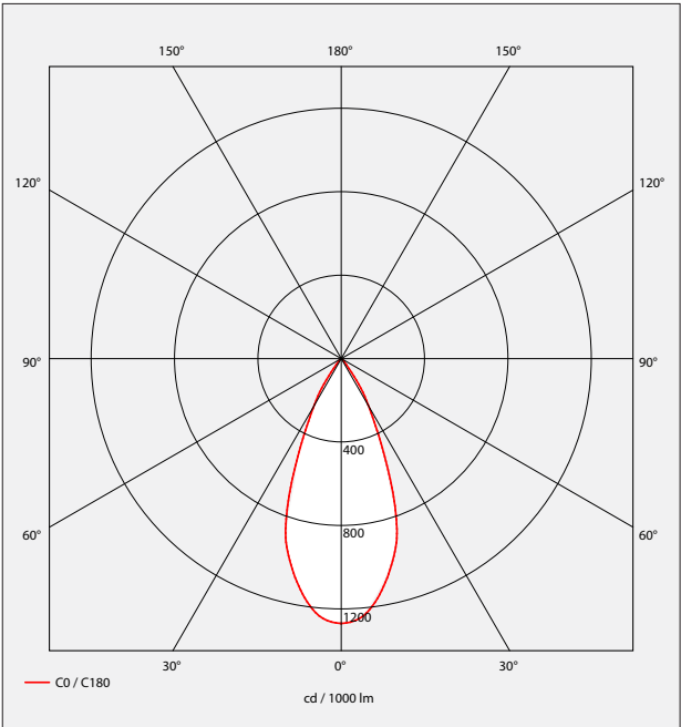
Beams 44° LOR 70,5%
