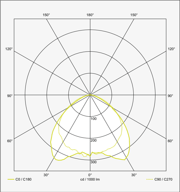
Optique Symétrique : Rendement 95 % SYM
