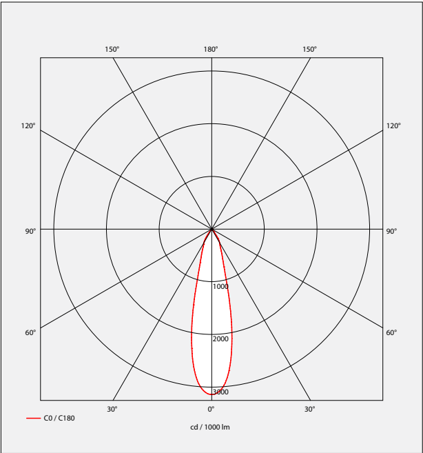
Faisceau 30° Rendement 88,8%
