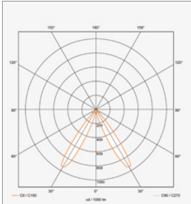
Réflecteur de type M8 haut* Rendement 90 %
