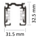
Rail Plafonnier
