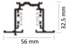
Rail Encastré
