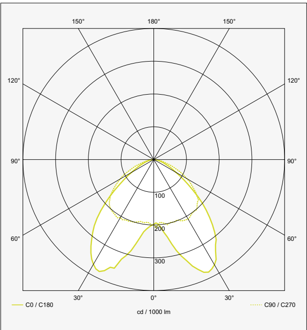
Optique Double Asymétrique : Rendement 95 % DASY
