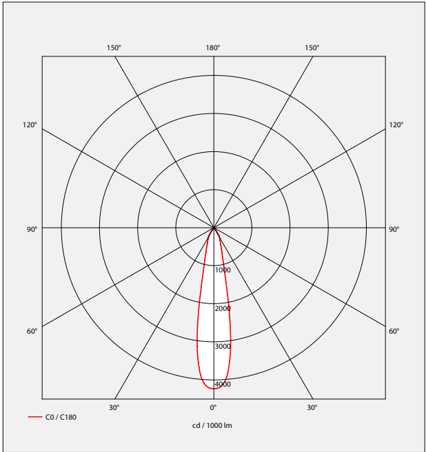
Faisceau 20° Rendement 90,8%
