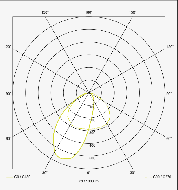
Optique Asymétrique : Rendement 91 % ASY
