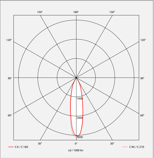
Faisceau 24°
