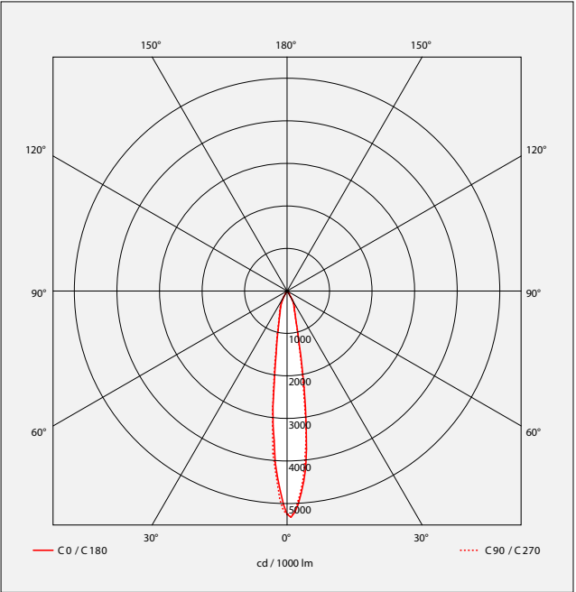
Faisceau 15°
