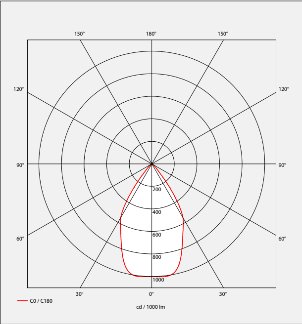
Beams 60° LOR 93,3%
