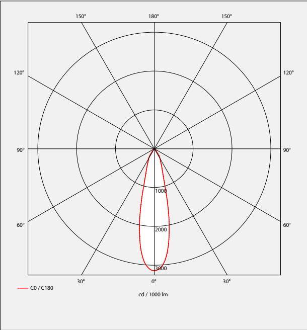
Faisceau 30° Rendement 78,8%
