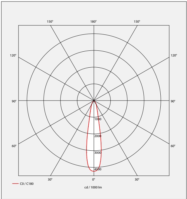
Faisceau 20° Rendement 90,8%
