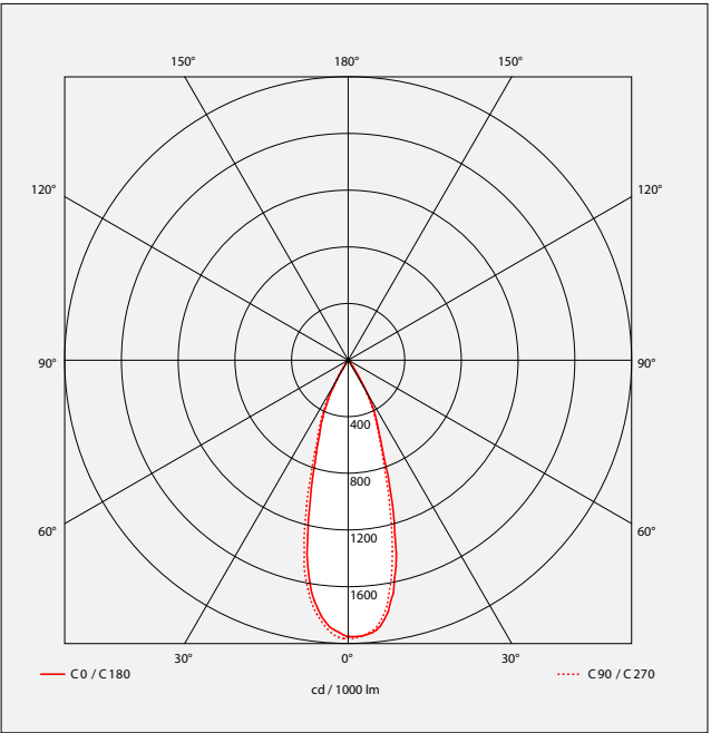
Faisceau 36°
