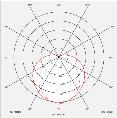
Longueur : 1198 mm
