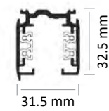
Rail Plafonnier
